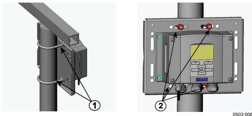
图 11 竖直支撑杆
