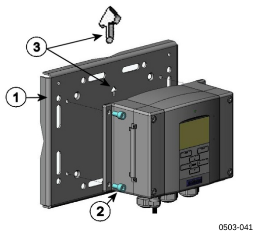
图 8 使用墙面安装金属板进行安装
