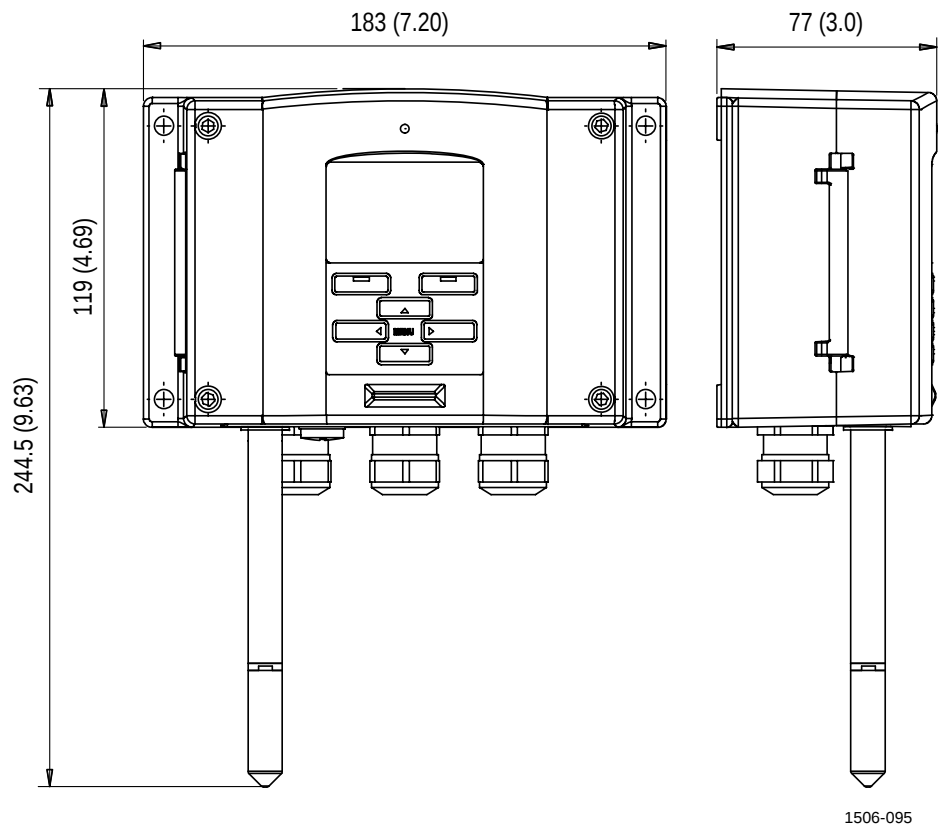
图 95 DMT341 尺寸
