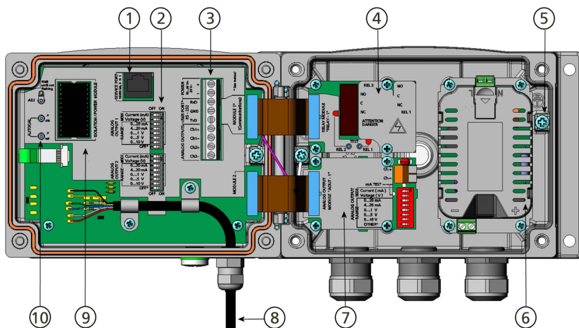
图 2 变送器内部
