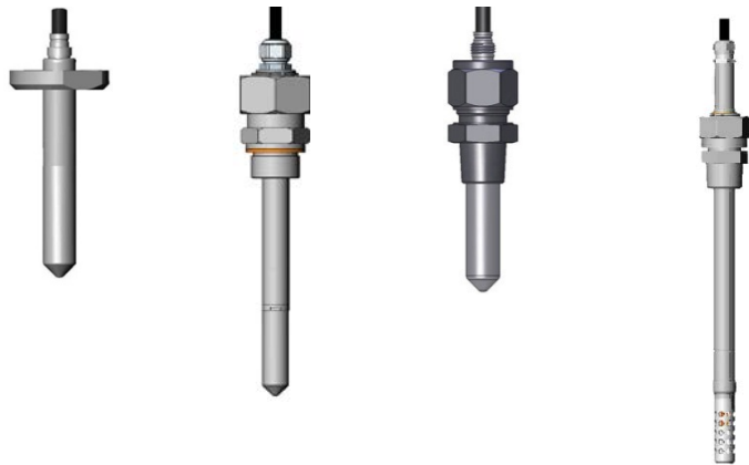
DMT342 小巧带法兰的探头，用于采样单元 用于高压应用的 DMT344 带 Swagelok 接头的 DMT347 探头 用于压力管路的 DMT348
