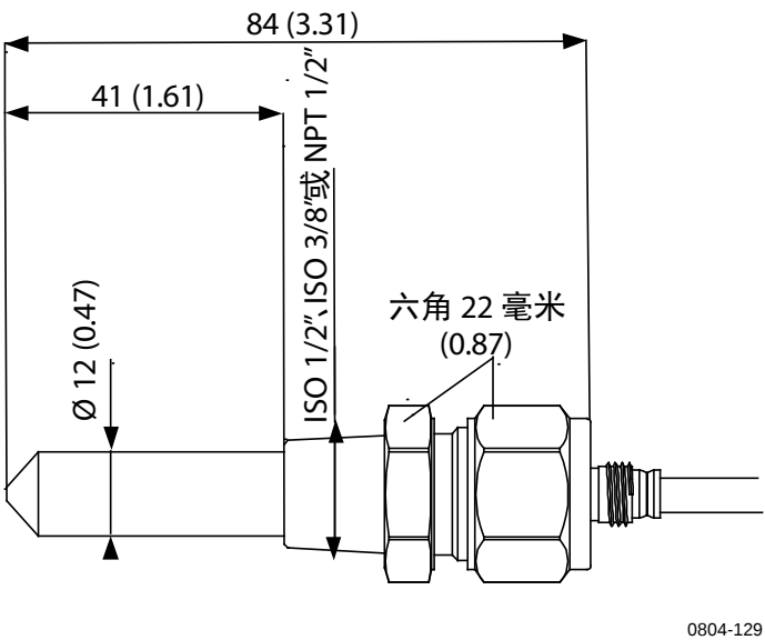
图 98 DMT347 探头尺寸
