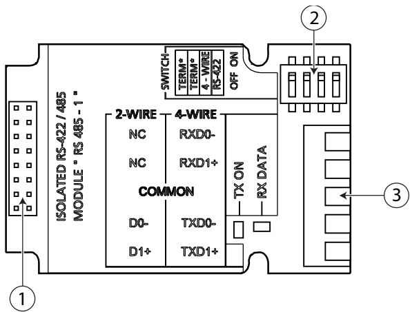
图 42 RS-422/485 模块
