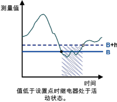
模式 2：仅设置了“低于”设置点
