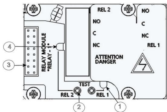
图 41 继电器模块
