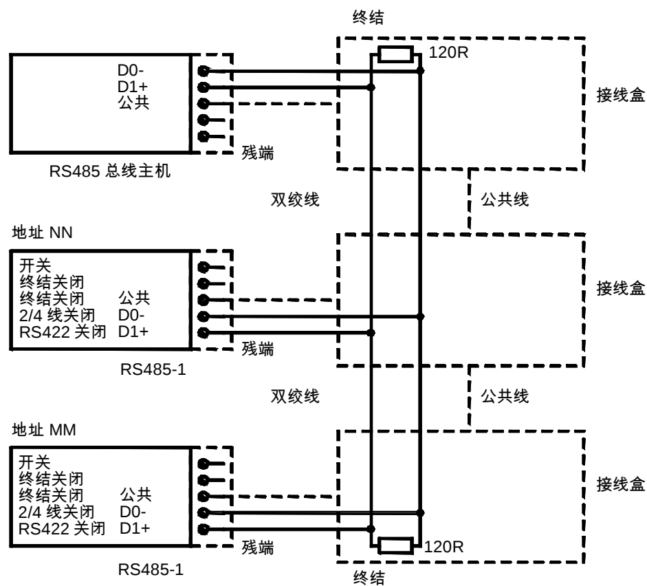
图 44 2 线 RS-485 总线
