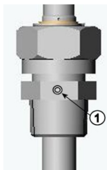
图 28 DMT348 探头中的放气螺钉
