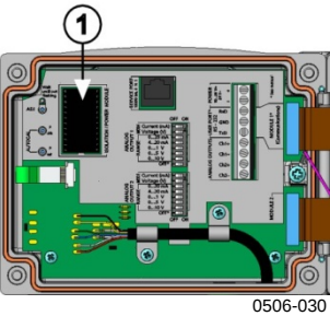
图 38 绝缘隔离模块
