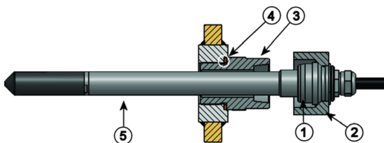
图 22 DMT344 探头
