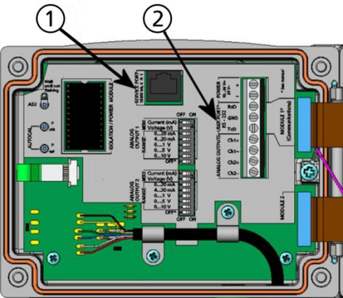
图 57 主板上的服务端口接头和用户端口终端
