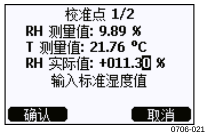
图 85 结束第 1 点的调校
