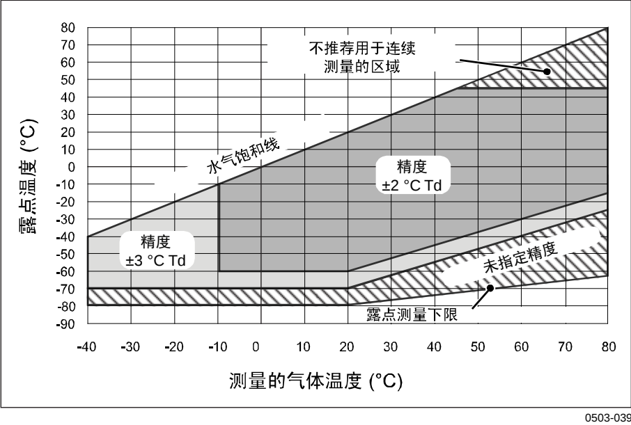
图 91 露点精度与测量条件
