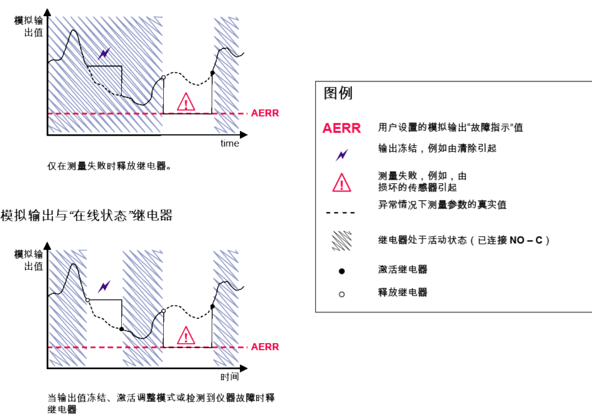
模拟输出与“故障状态”继电器
