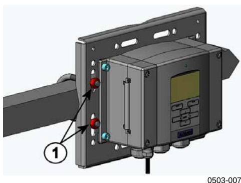
图 12 水平支撑杆
