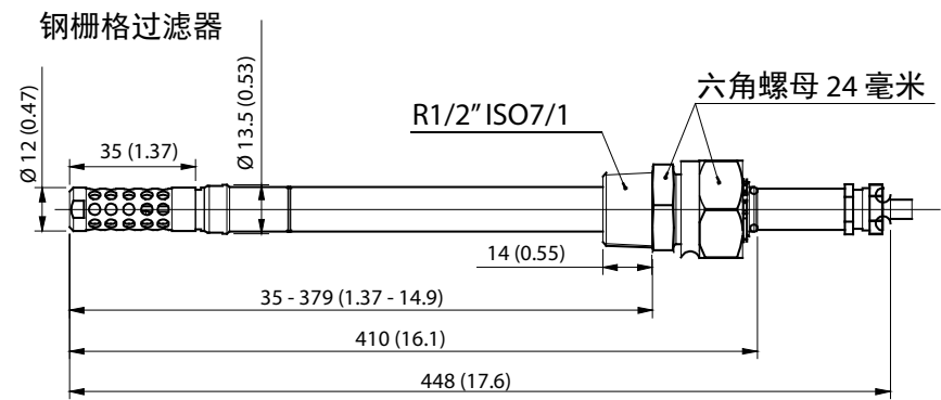
图 101 DMT348 可选的 400 毫米探头尺寸
